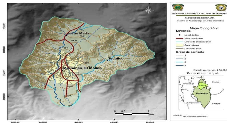
Figura 2. Topografía del Valle de Malinalco
