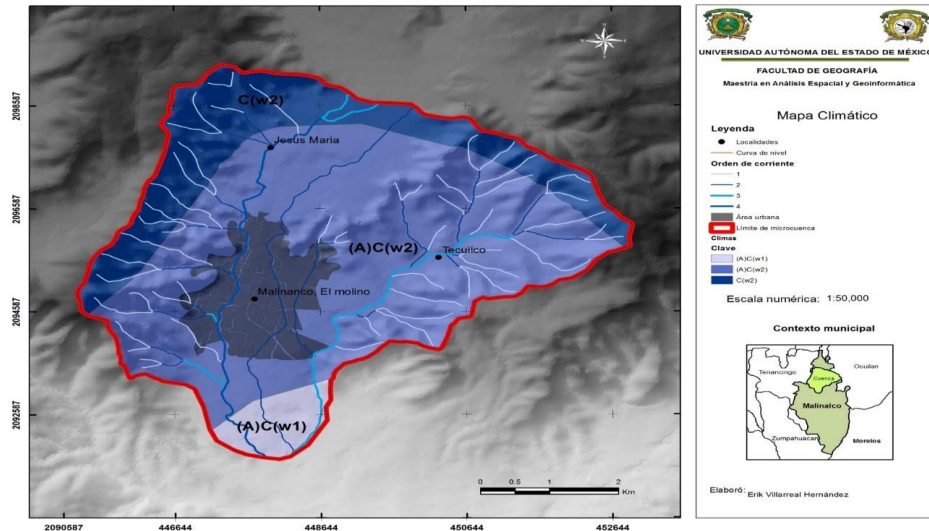
Figura 3. Climas del Valle del Malinalco
