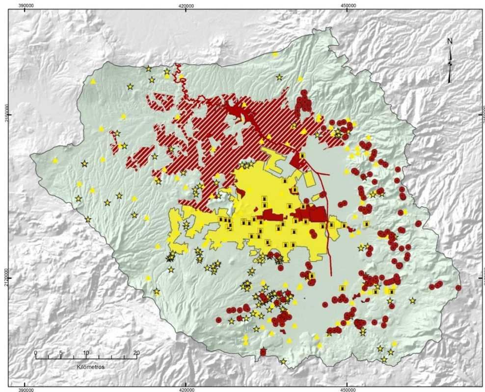
Figura 3.- Clasificación de fuentes de contaminación en el acuífero del Valle de Toluca
